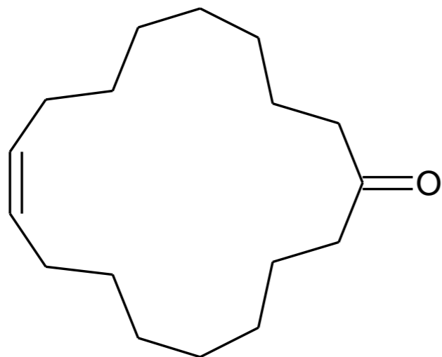
ジャコウネコの分泌物シベットの成分
