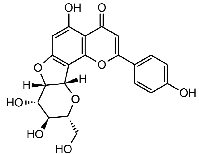
ウーロン茶成分
